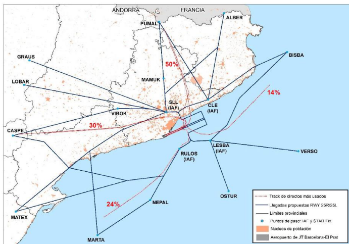
Figura 13. Previsión de directos en las llegadas por la RWY25R/L de LEBL recogida en el Documento Ambiental del proyecto BRAIN fase II. Fuente: ENAIRe.
