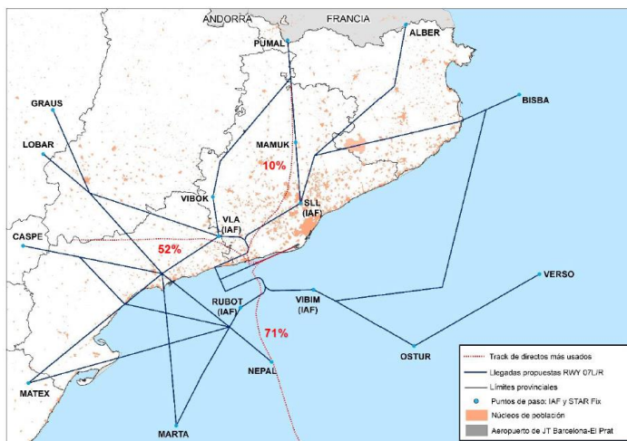
Figura 14. Previsión de directos en las llegadas por la RWY07R/L de LEBL recogida en el Documento Ambiental del proyecto BRAIN fase II. Fuente: ENAIRe.
