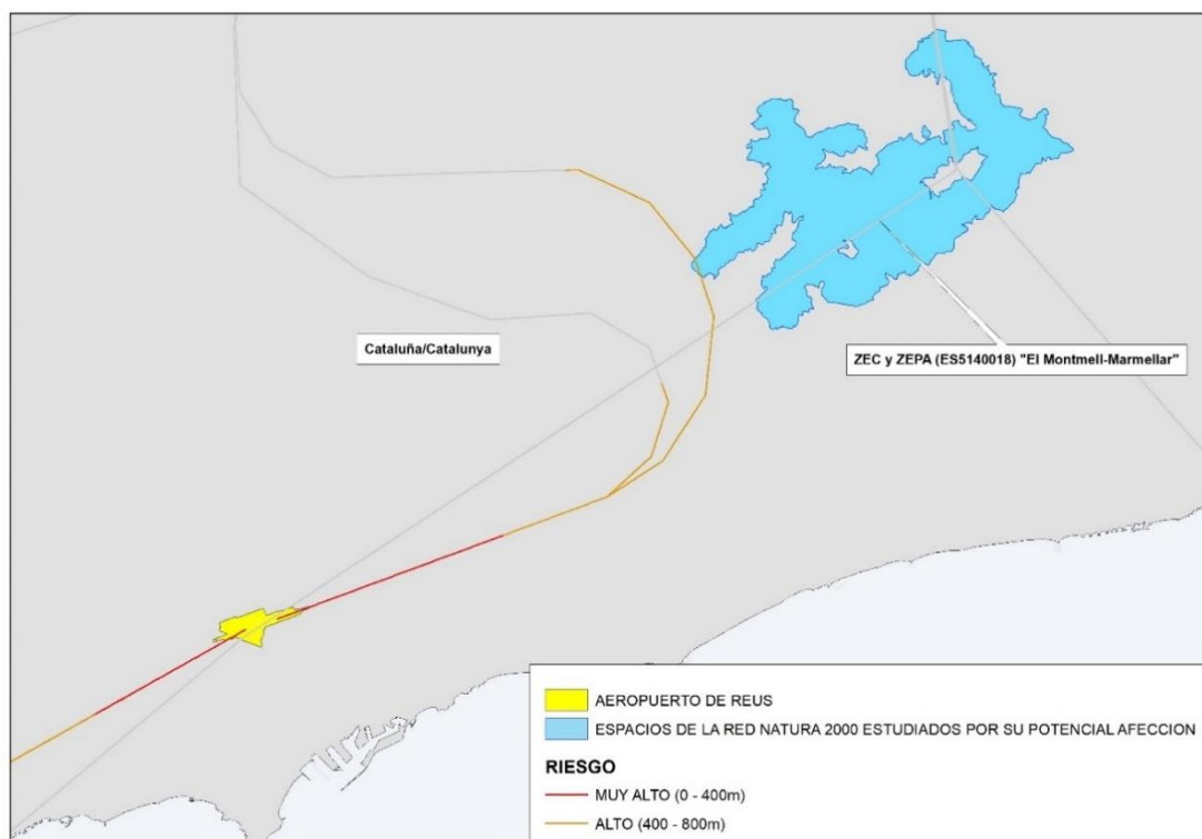
Figura 7. Sobrevuelo de las maniobras de salida a través de la cabecera 07 sobre el espacio de la Red Natura 2000 ZEC y ZEPA “El Montmell-Marmellar”. Fuente: elaboración propia.
