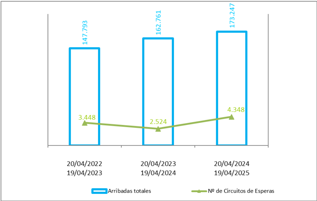
Figura 2. Números de circuitos de esperas frente al número total de llegadas en el Aeropuerto de Josep Tarradellas Barcelona-El Prat frente a los períodos considerados.
